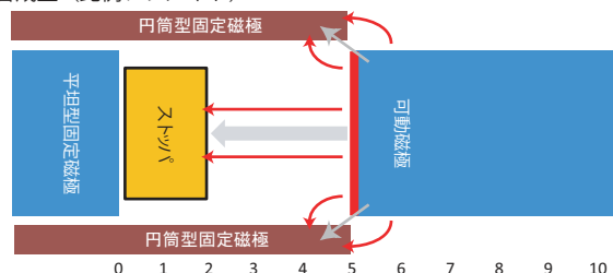
図1 各種ソレノイドの磁極と特性
