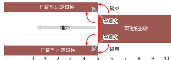
合成型 (比例ソレノイド)
